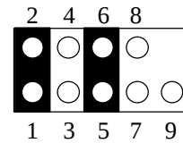
Cable Select
